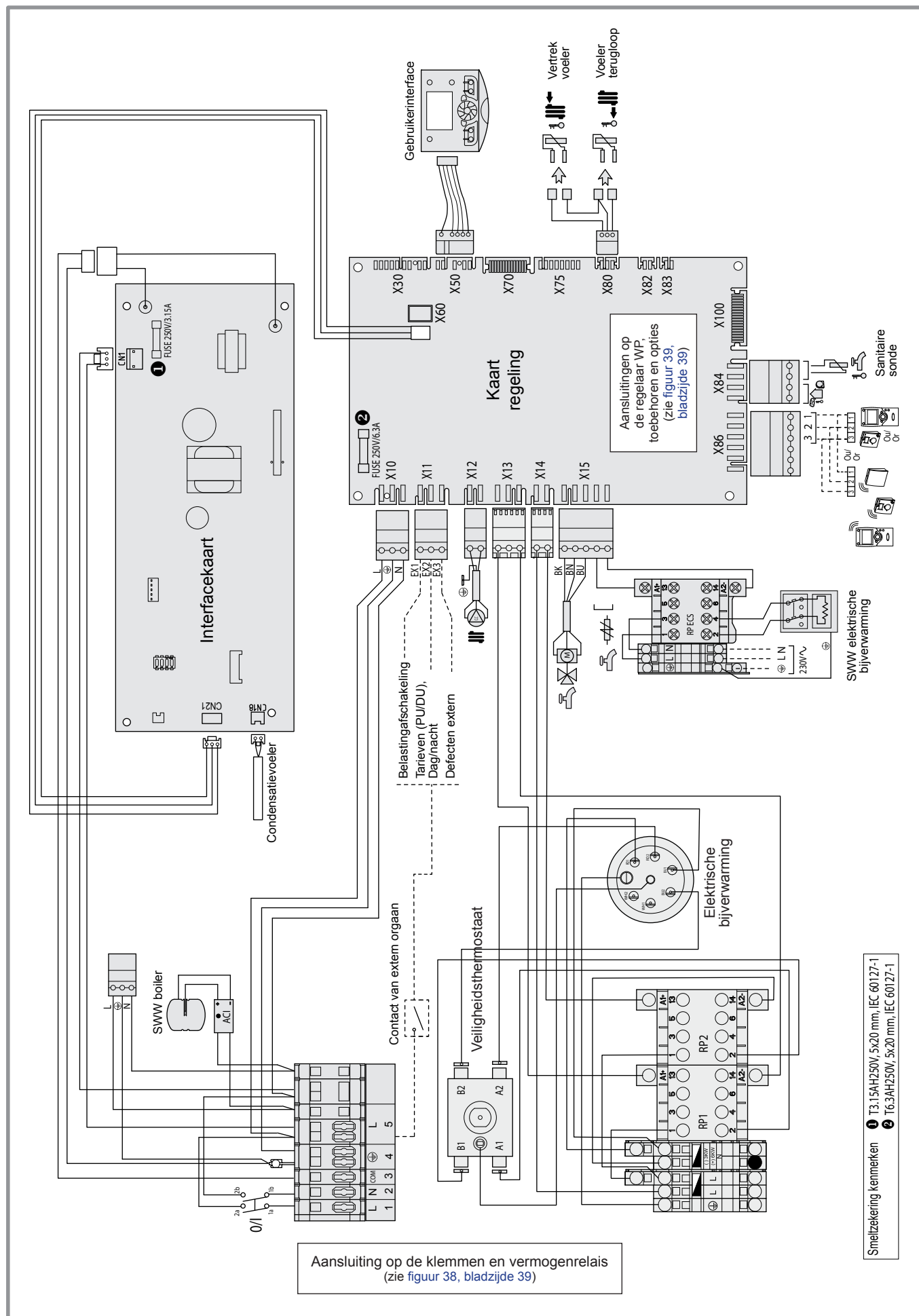
figuur 49 - Elektrisch kablering, Hydraulische module (Behalve aansluitingen door de installateur)
