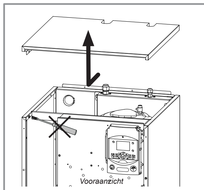
figuur 16 - Afnemen van het deksel
