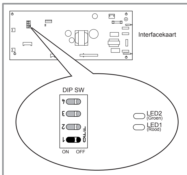
figuur 23 - Plaats van de DIP-schakelaars en de LED op de interfacekaart van de hydraulische module.
