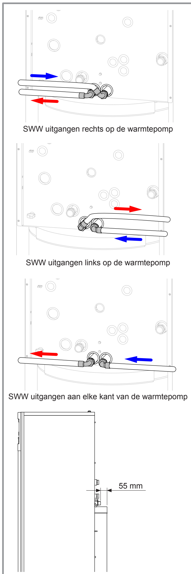
figuur 26 - SWW uitgangen
