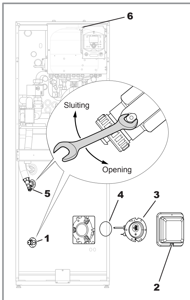
figuur 50 - De hydraulische module ledigen en/of Sanitaire boiler
