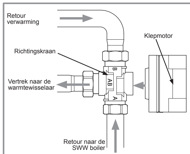
figuur 51 - Montage van de richtingsklep
