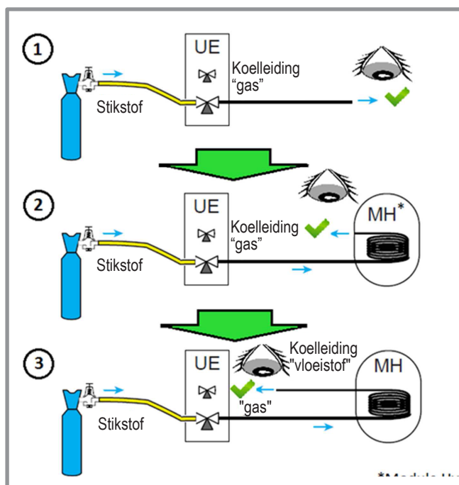
figuur 19 - Contrôle van de koeltechnische leidingen
