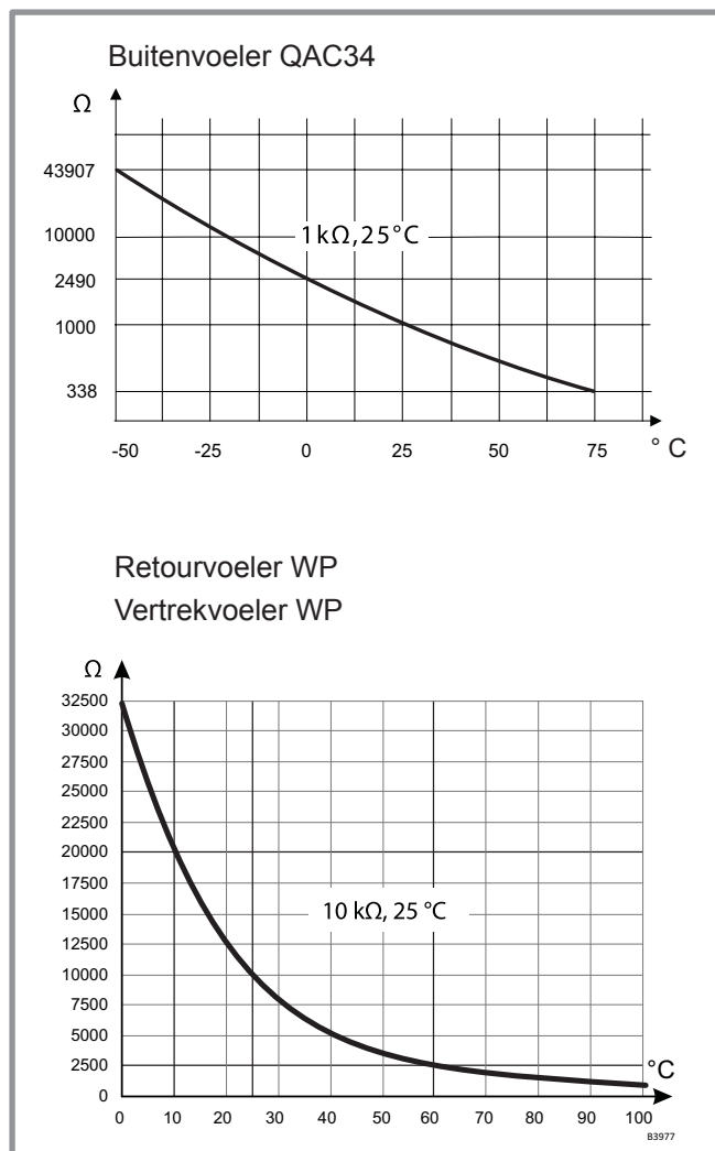
figuur 4 - Waarde in ohm van de voelers (Hydraulische module)
