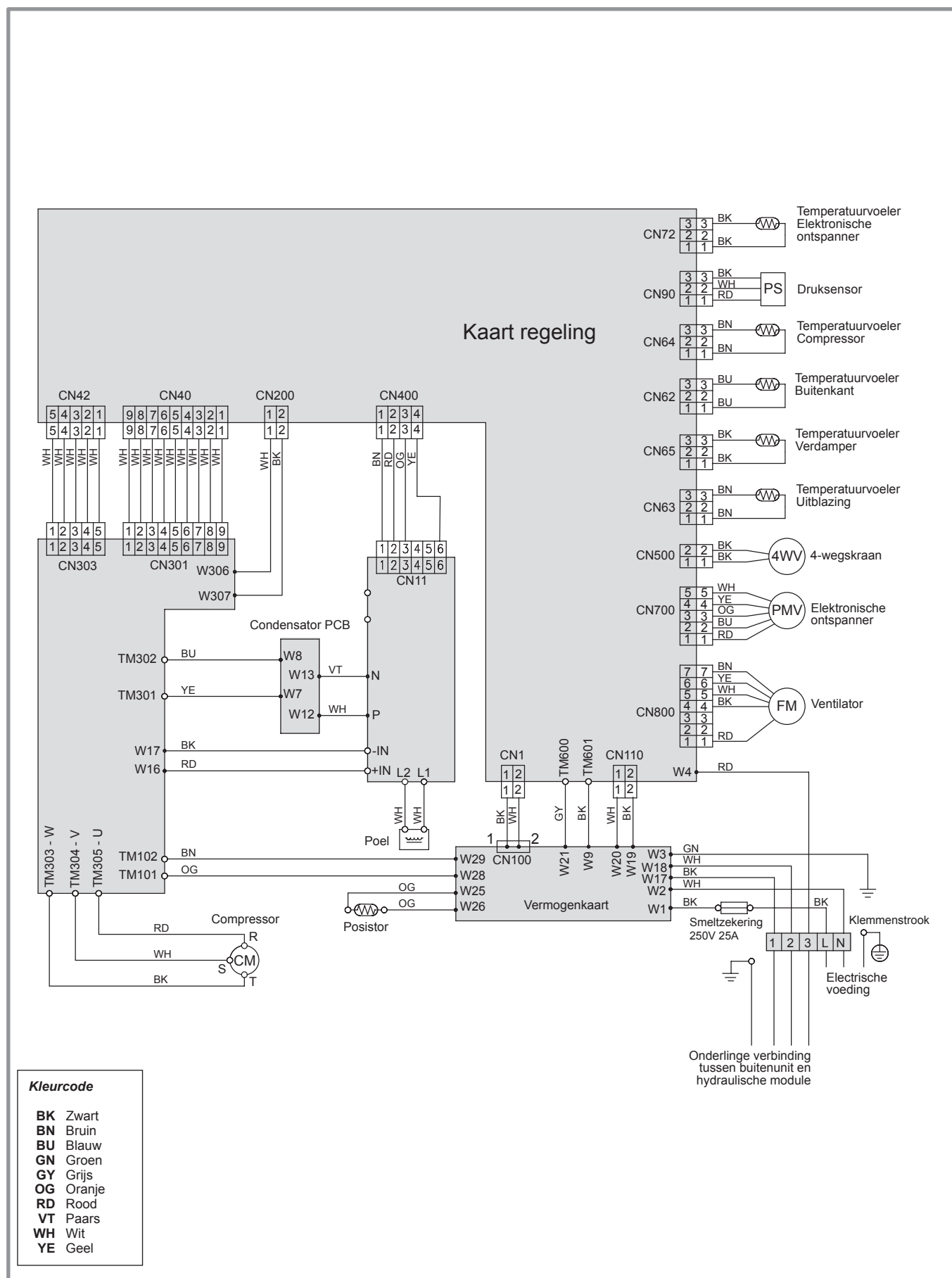
figuur 48 - Elektrisch kablering buitenunit model Comfort 10
