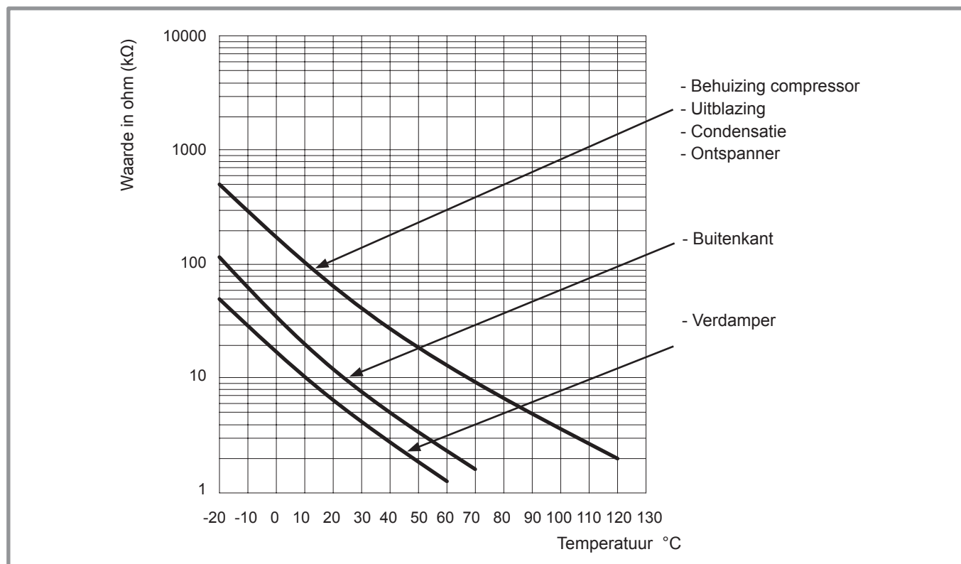
figuur 5 - Waarde in ohm van de voelers (Buitenunit)
