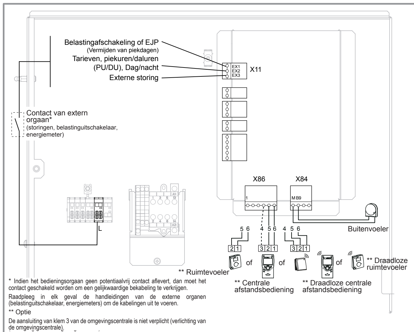
figuur 39 - Aansluitingen op de regelaar WP (toebehoren en opties)
