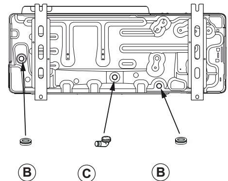
figuur 13 - Plaatsing van de buitenunit, afvoer van de condensaten
