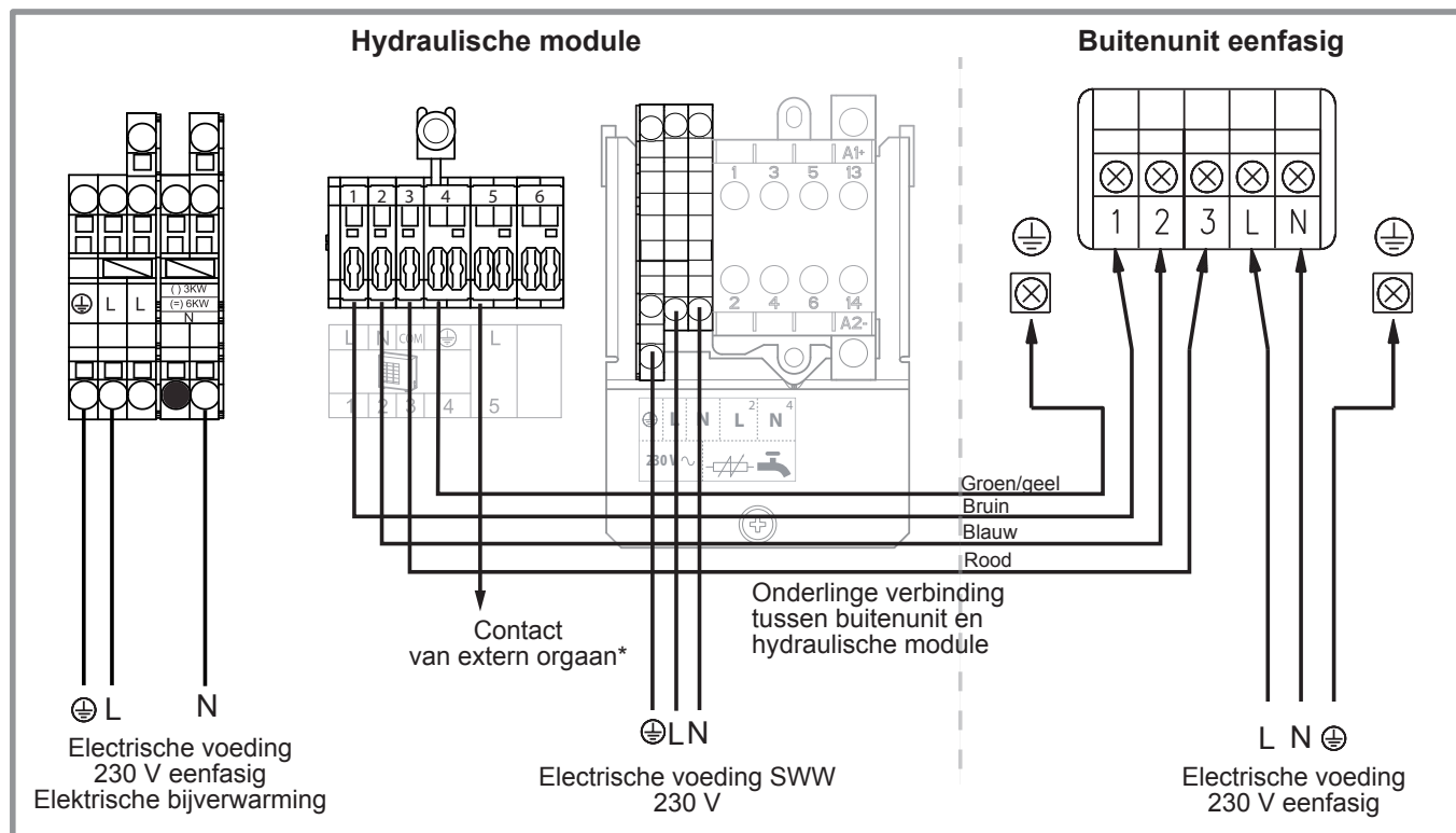
figuur 38 - Aansluiting op de klemmen en vermogenrelais
