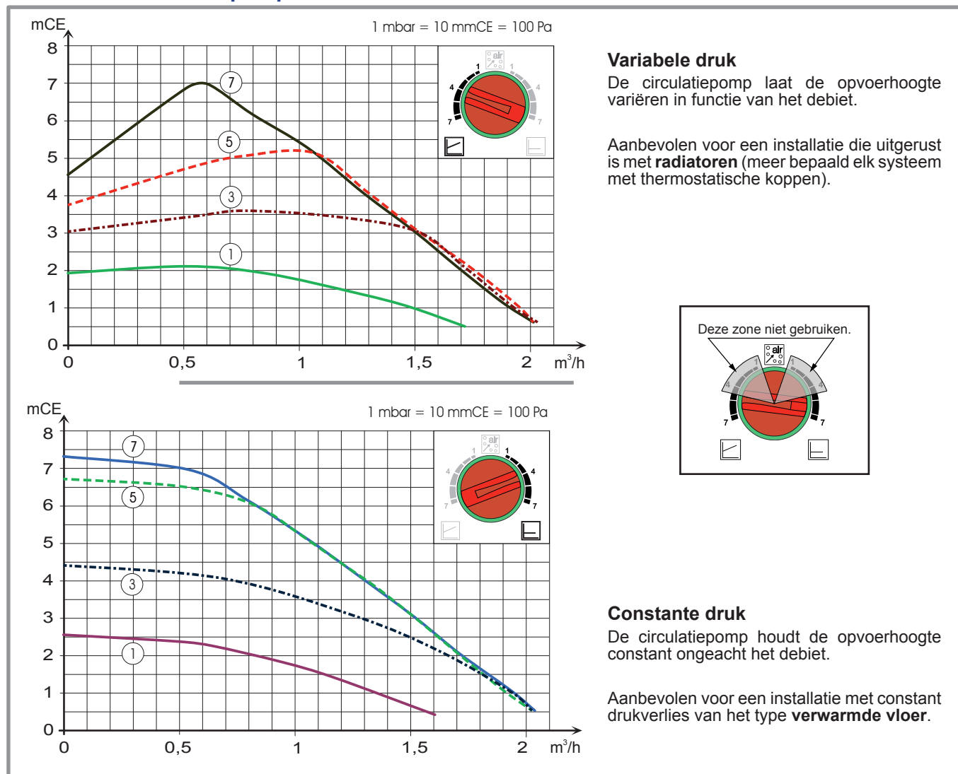
figuur 30 - Beschikbare drukken en hydraulische debieten
