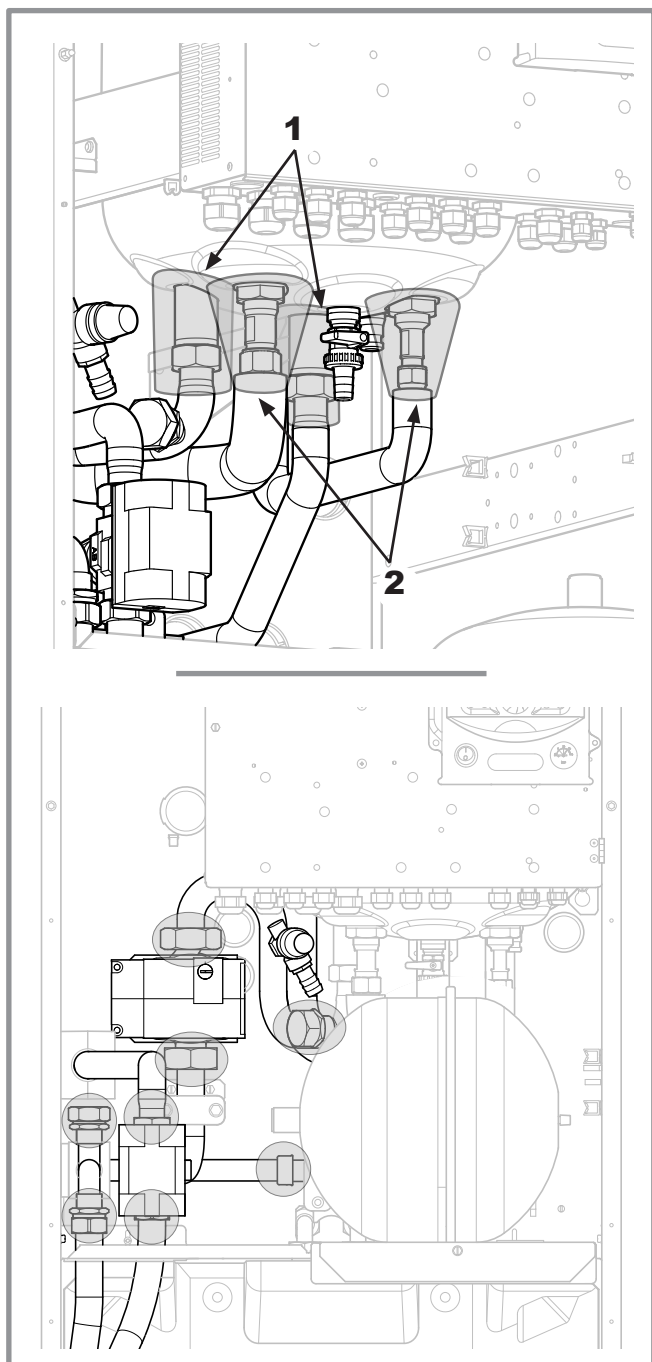
figuur 29 - Thermische isolatie
