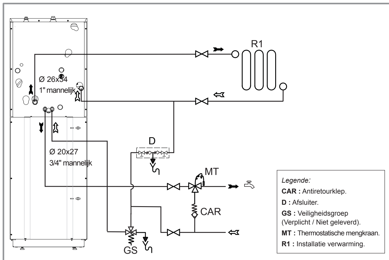
figuur 24 - Principieel hydraulisch schema
