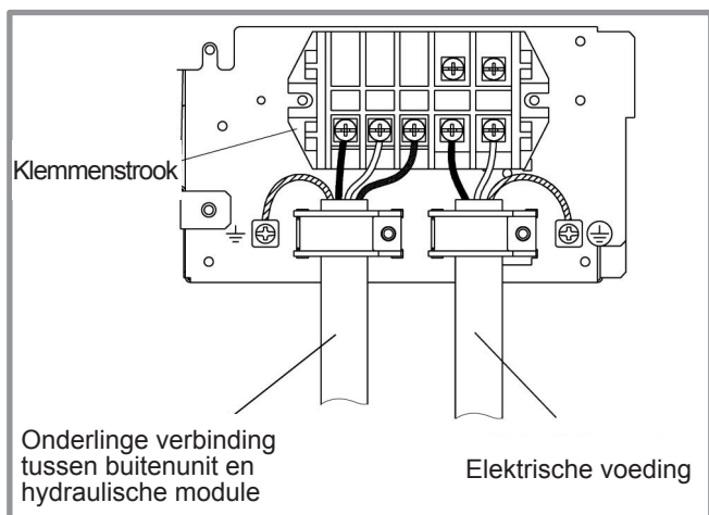
figuur 34 - Aansluitingen op de klemmenstrook van de buitenunit
