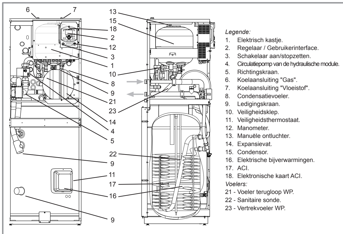
figuur 7 - Organen van de hydraulische module
