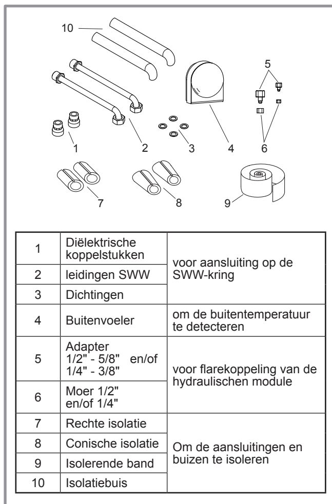
figuur 10 - Met de hydraulische module geleverd toebehoren
