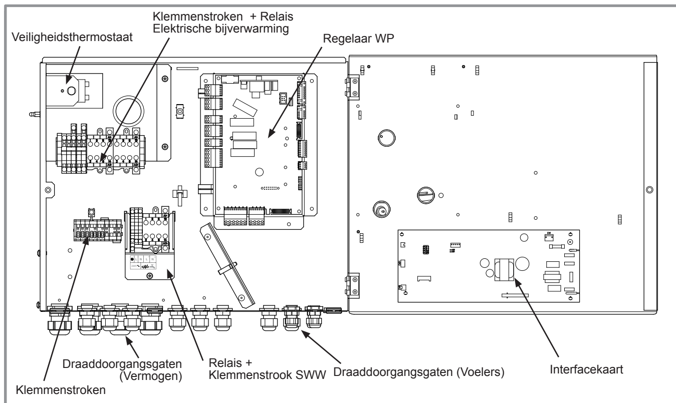
figuur 37 - Toegang tot het elektriciteitskastje van de hydraulische module en beschrijving
