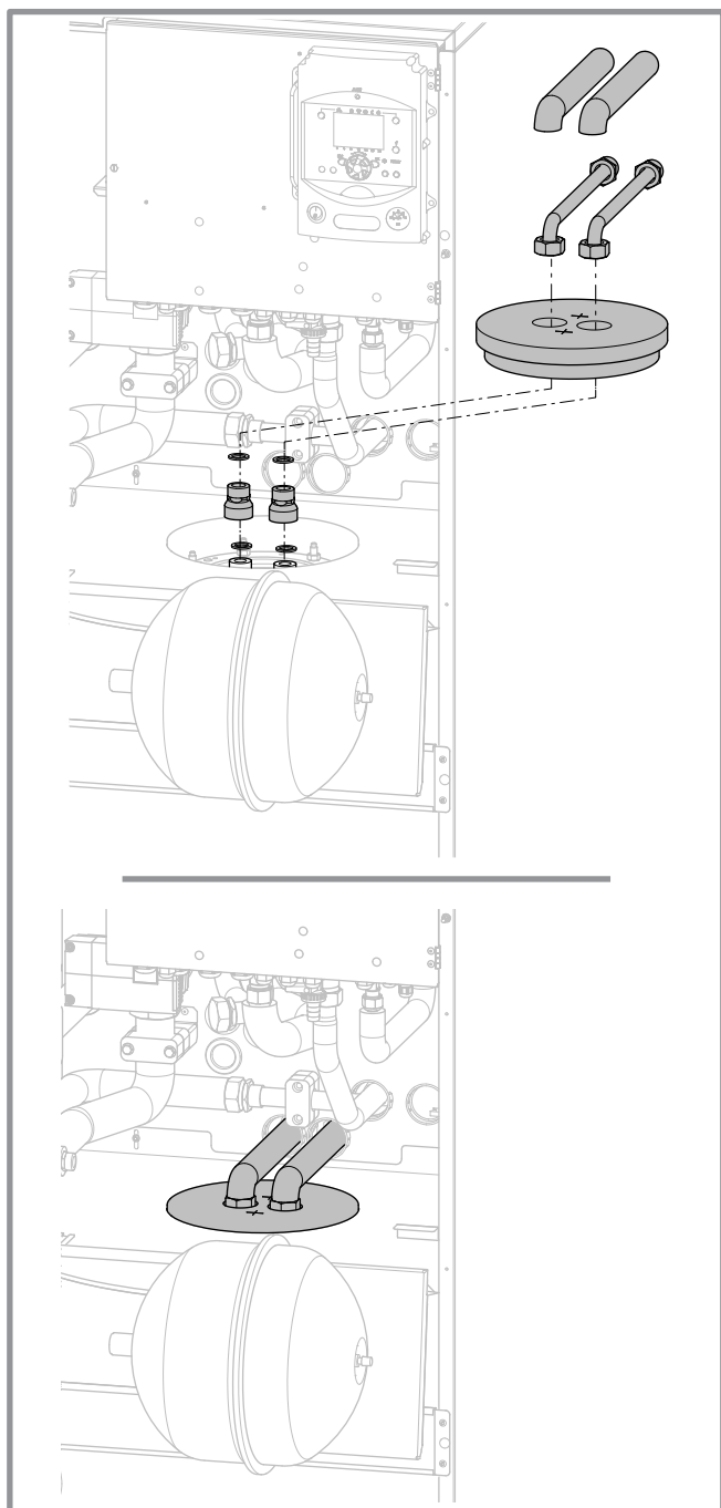
figuur 25 - Aansluiting van de SWW leidingen
