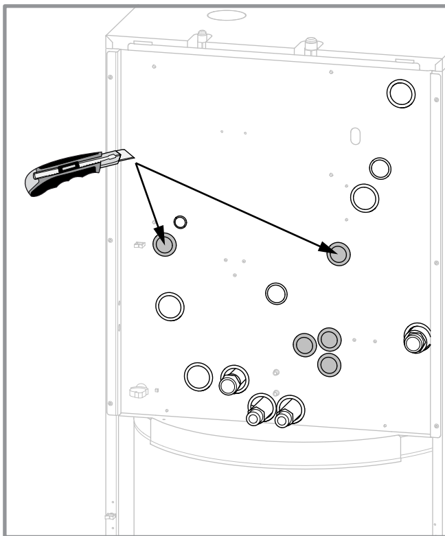
figuur 36 - Doorgang van de kabels langs de achterkant van de hydraulische module
