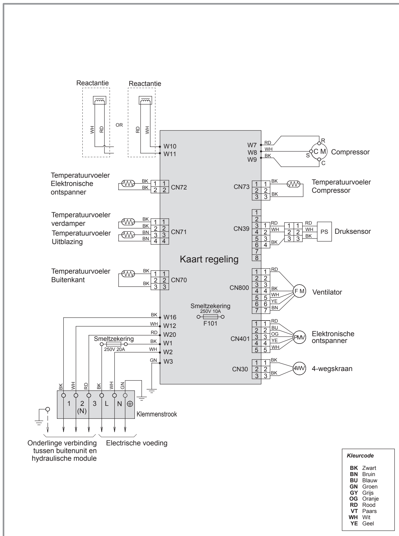
figuur 46 - Elektrisch kablering buitenunit model Comfort 5 en 6
