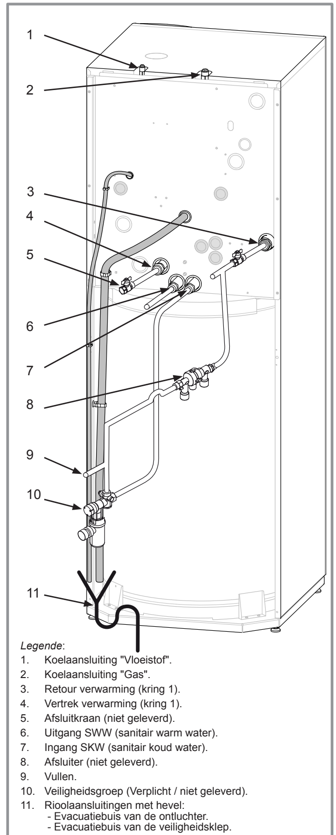
figuur 28 - Aansluitingen
