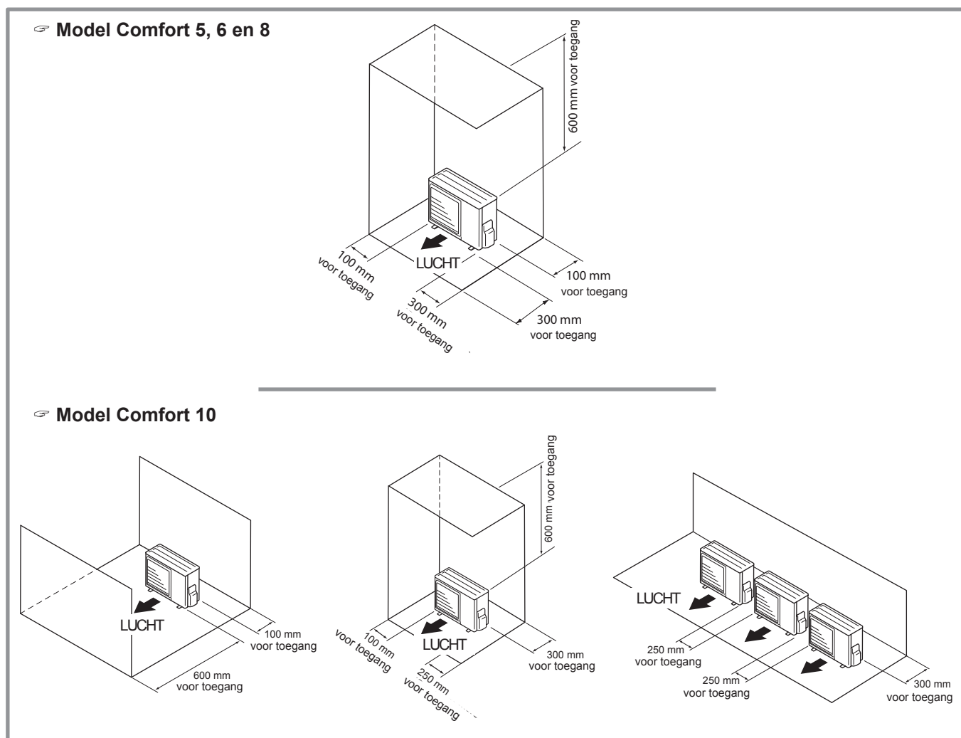
figuur 12 - Minimale installatieruimte rondom de buitenunit (Alle modellen)
