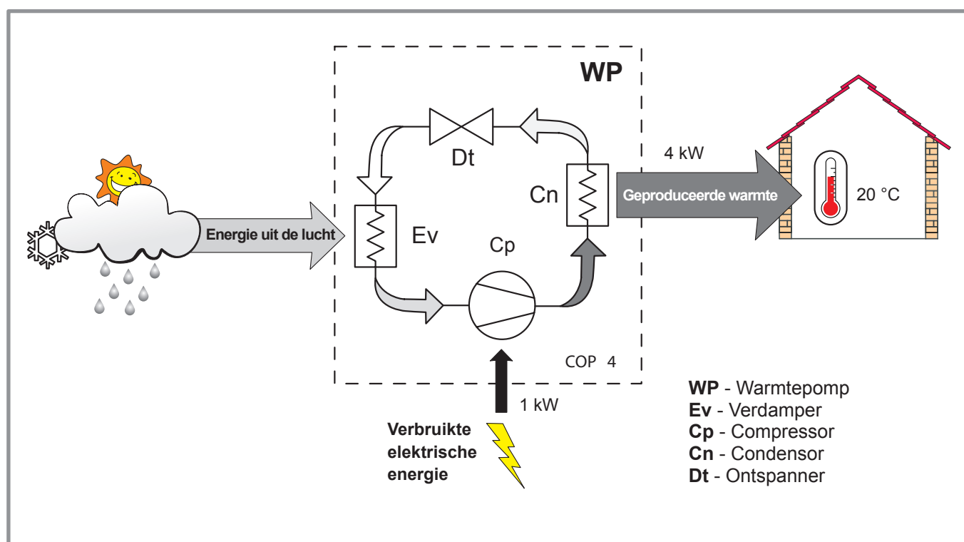
figuur 8 - Weringsprincipe van een warmtepomp
