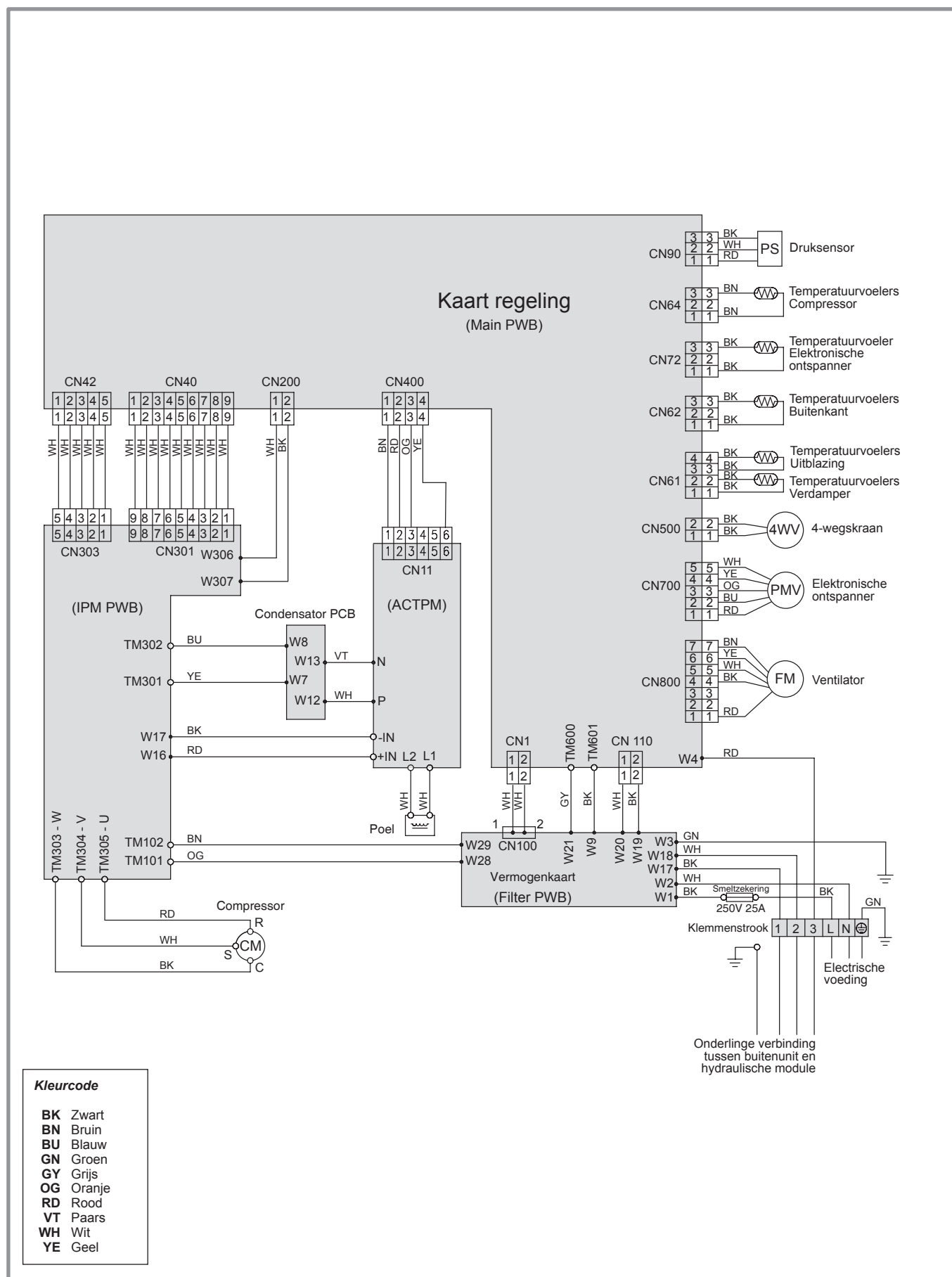
figuur 47 - Elektrisch kablering buitenunit model Comfort 8
