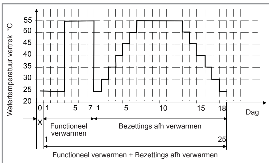
figuur 45 - Diagramma van de droogprogramma's voor vloerplaten
