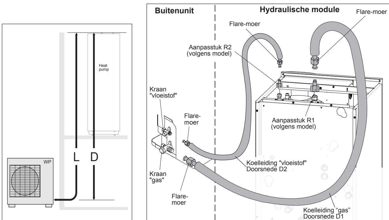
figuur 20 - Koelverbindingen Aansluiting (Diameters en toegelaten lengten)
