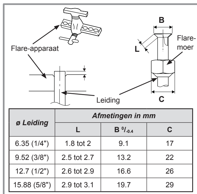
figuur 17 - Verwijding voor flareverbindingen
