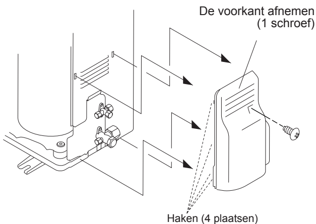
figuur 35 - Toegang tot de klemmenstrook van de buitenunit
