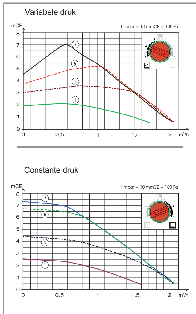
figuur 3 - Beschikbare drukken en hydraulische debieten
